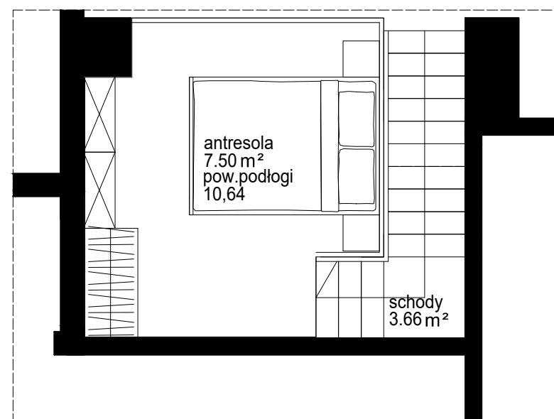
RZUT ANTRESOLI
