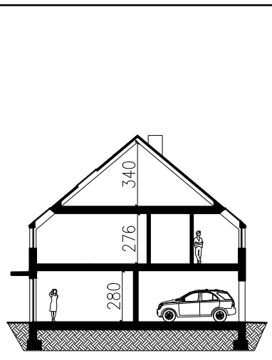
SCHEMAT PRZEKROJU
