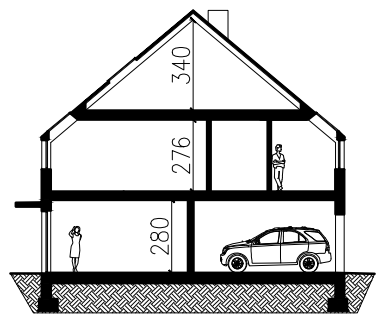
SCHEMAT PRZEKROJU
